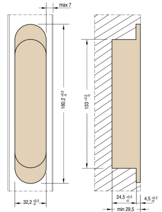
Cutout dimension 開槽尺寸
