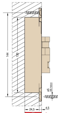
Hinge dimensions 鉸鏈尺寸
