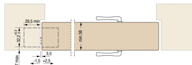
Hinge dimensions 鉸鏈尺寸
