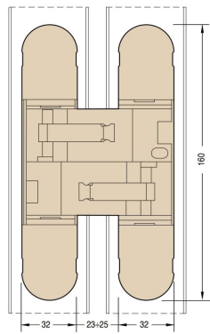
Hinge dimensions 鉸鏈尺寸
